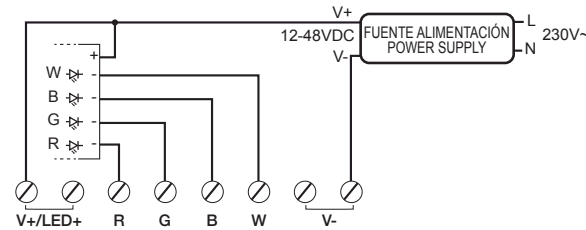
Regulación de Tira RGB / RGBW LED Strip Dimming
